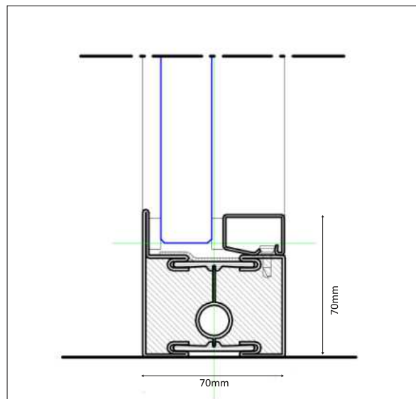
IQ-PROTECT EI60 profiel doorsnede
