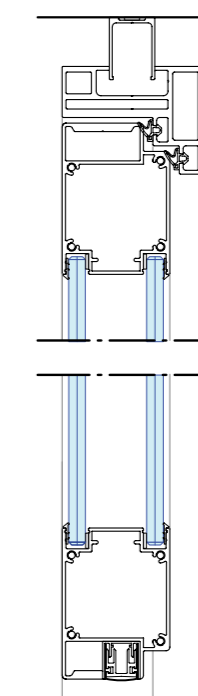
KDD57D - DK74D verticale doorsnede
